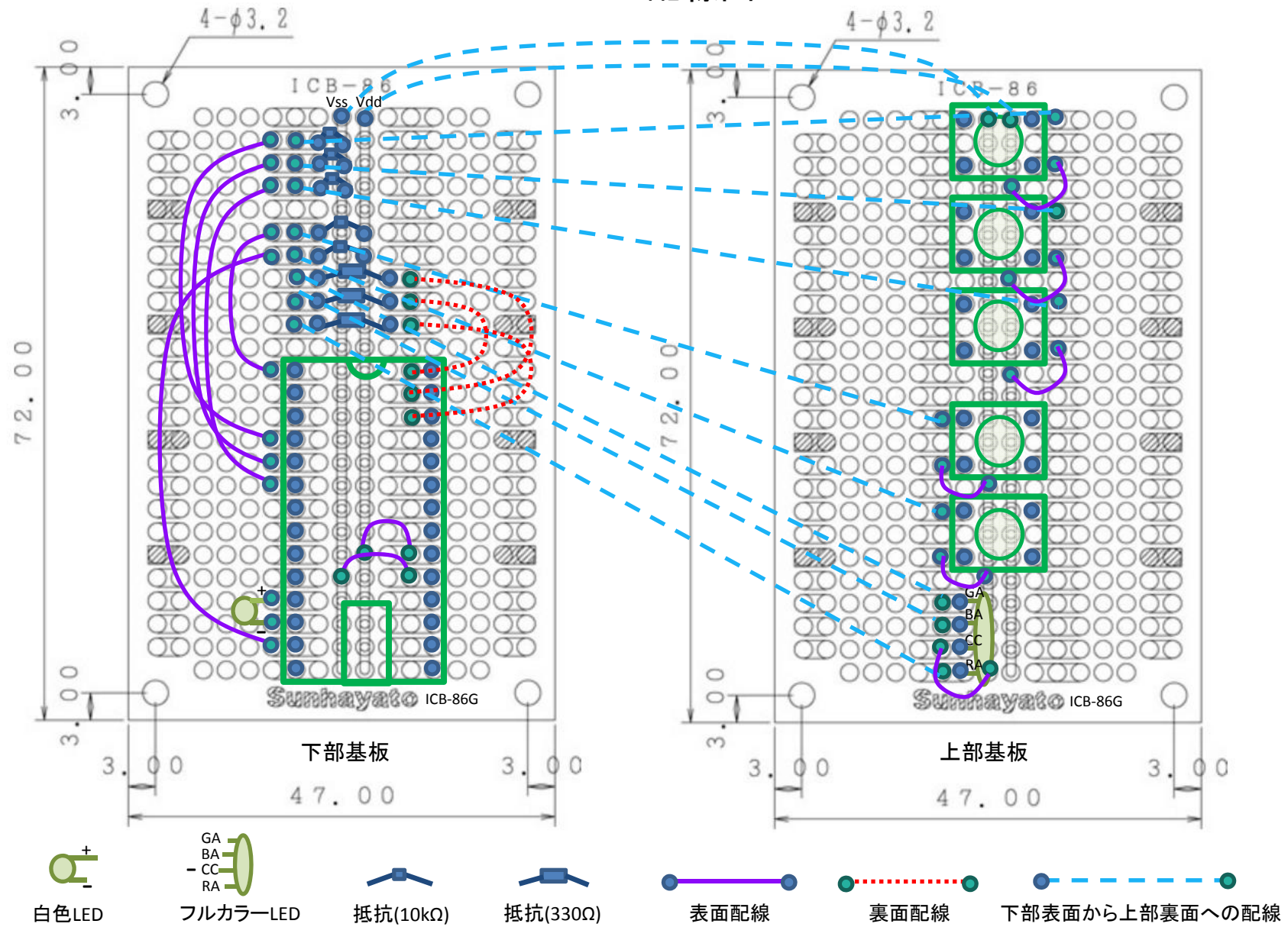
PIC-GPE配線図
